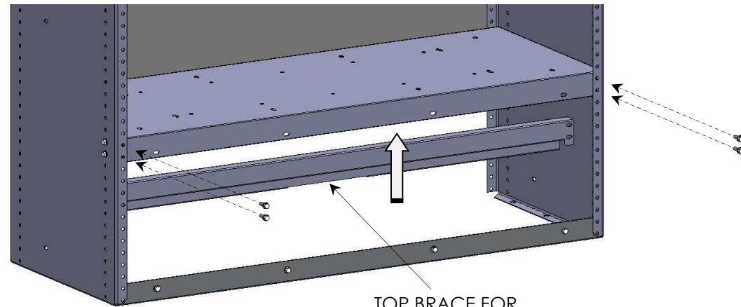
TOP BRACE FOR FLUSH MOUNT DOOR
